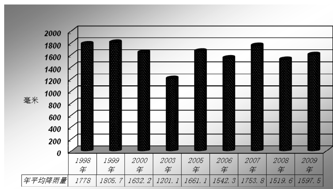
1998 年-2009 年浙江省平均降雨量
