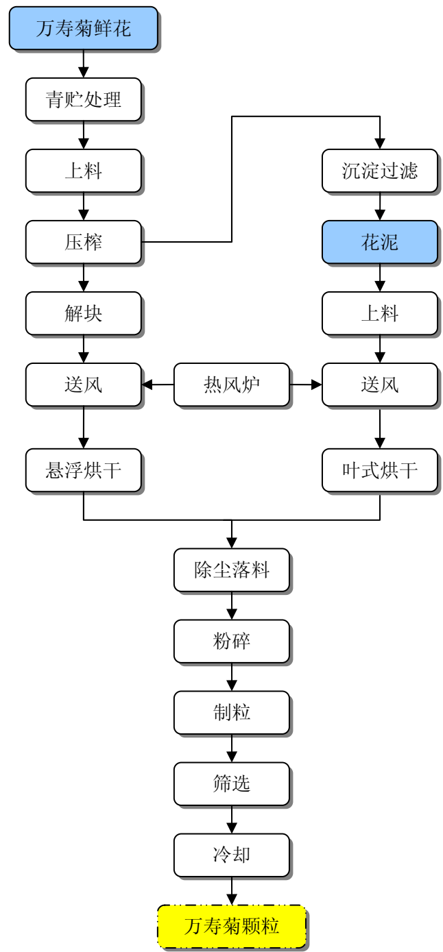
图 6-8 万寿菊颗粒生产工艺流程图
