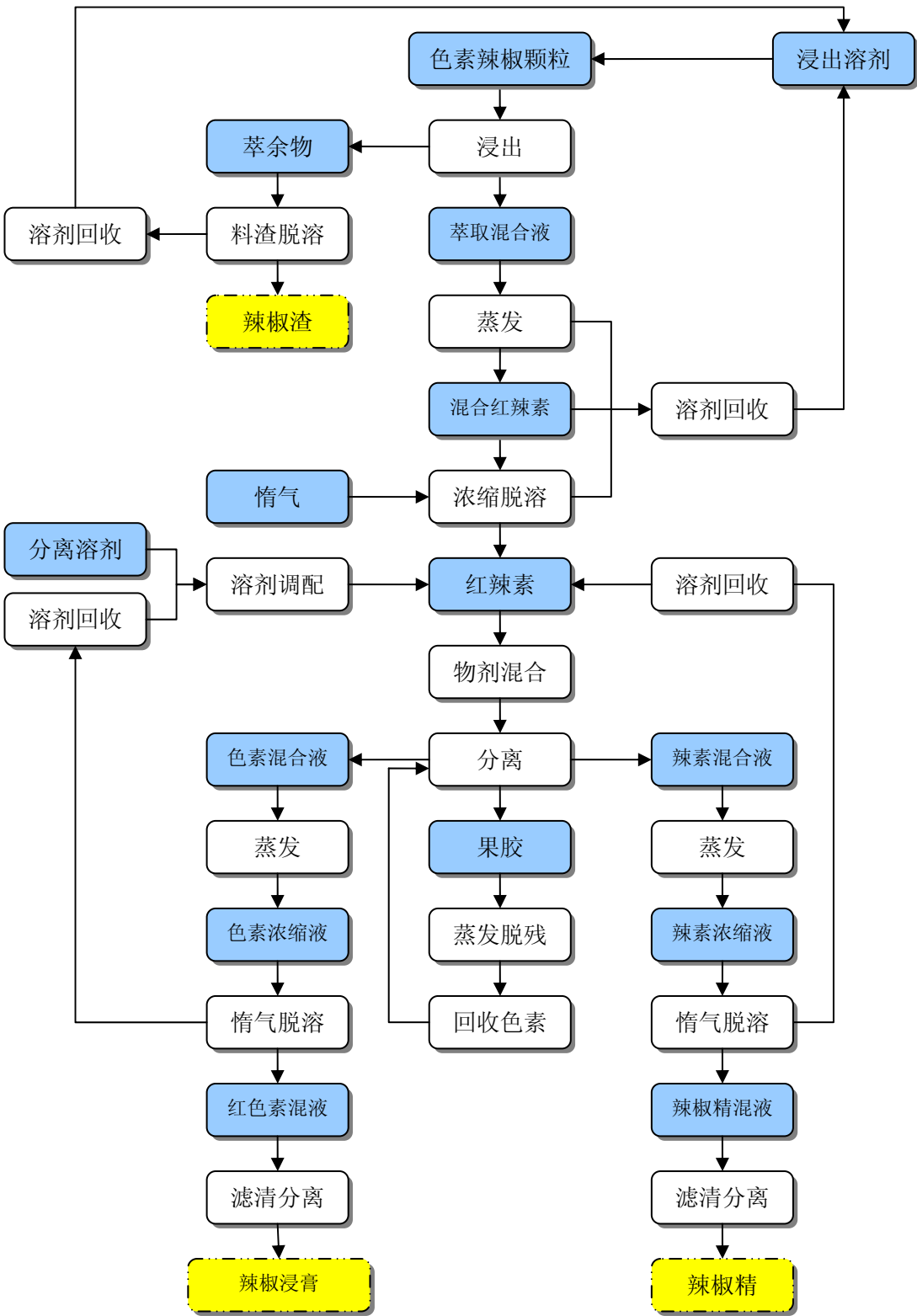
图 6-11 辣椒浸膏生产工艺流程图
