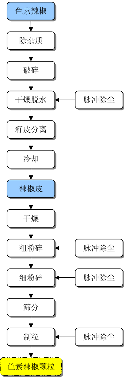
图 6-10 色素辣椒颗粒生产工艺流程图
