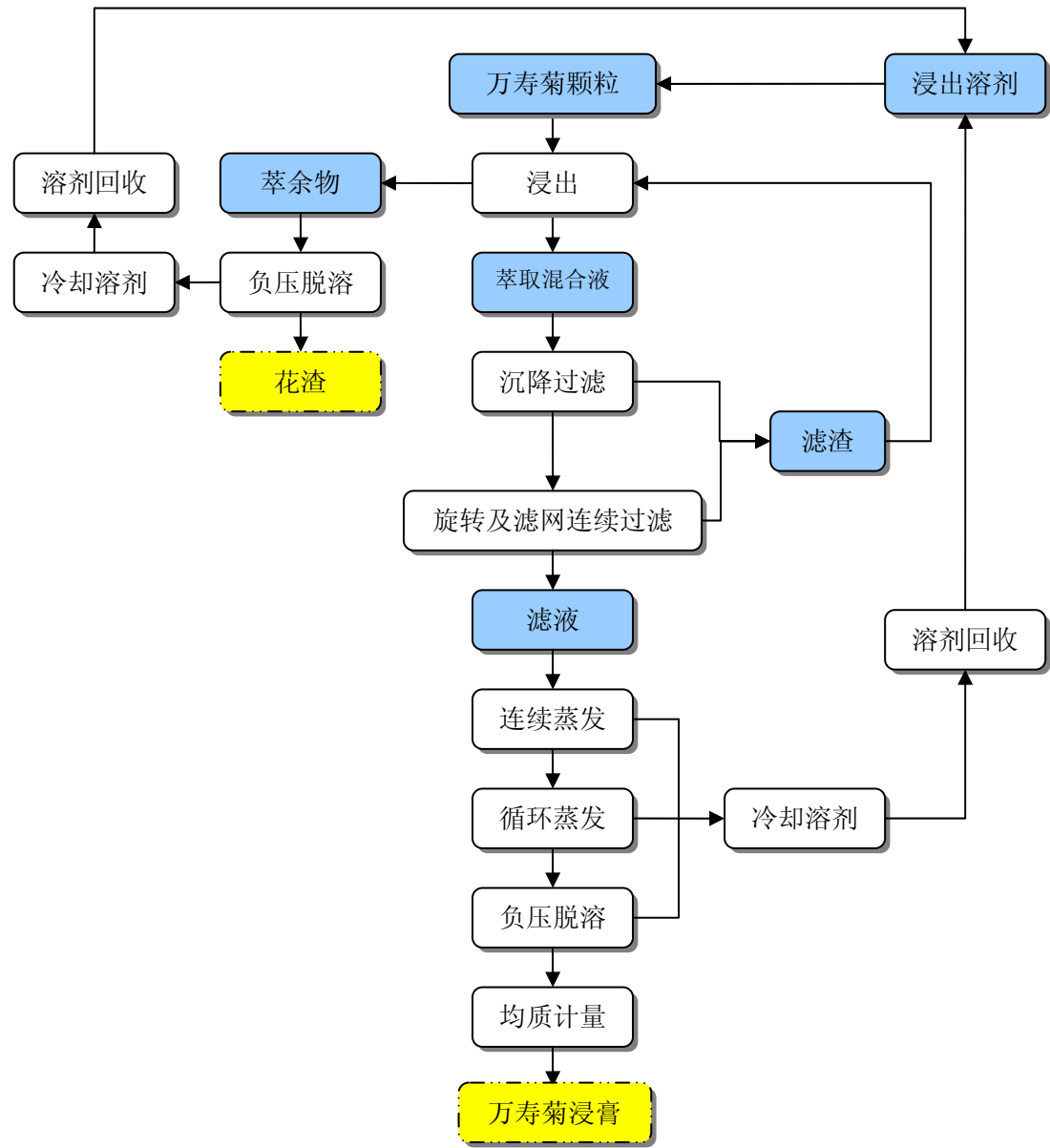
图 6-9 万寿菊浸膏生产工艺流程图
