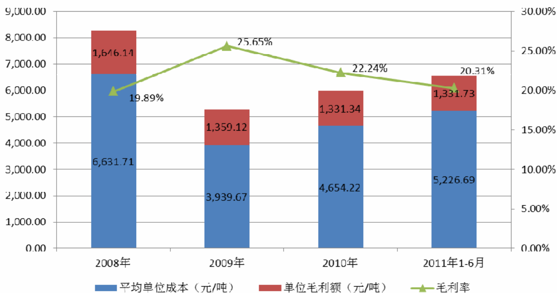
直缝埋弧焊接钢管毛利率变动情况
