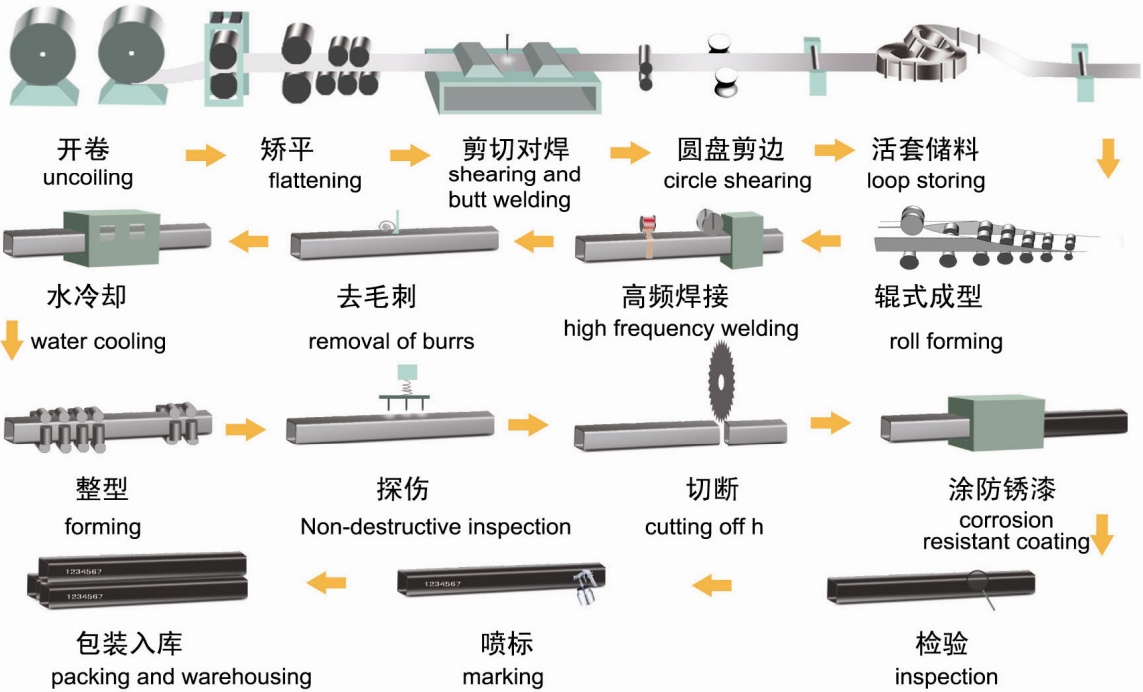
矩形钢管生产工艺流程图
