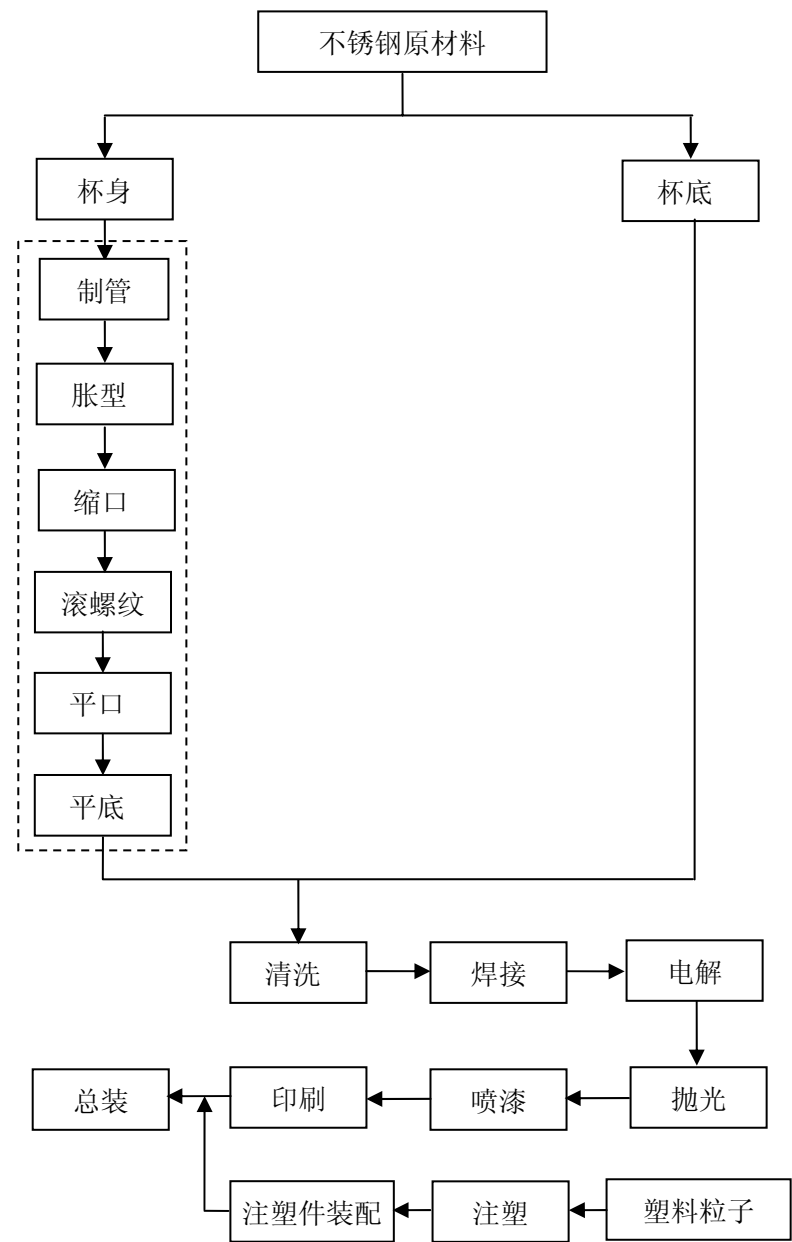
不锈钢非真空器皿工艺流程图
