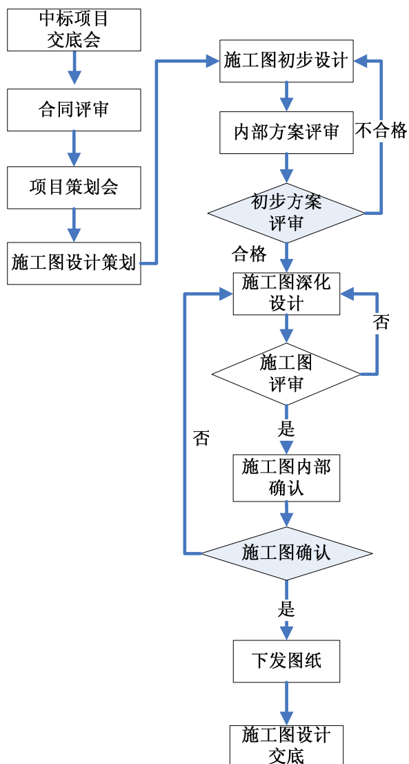
b. 施工图设计流程
