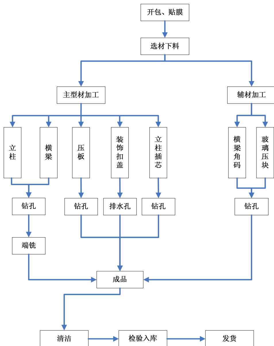
构件式（半隐框幕墙）加工工艺流程图：
