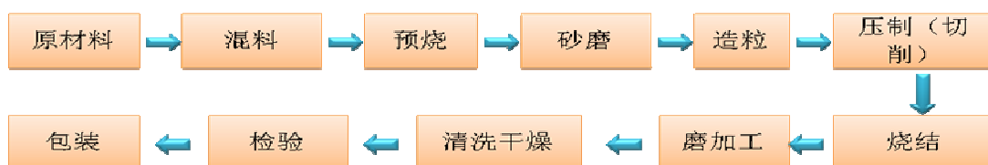
(2) 镍锌软磁铁氧体工艺流程图
