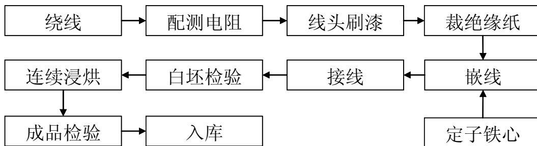
成品定子生产工艺流程图
