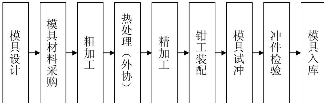
模具加工工艺图
