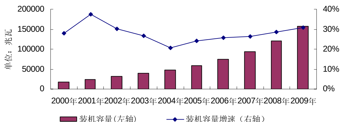
2000年—2009年全球风电累计装机容量及增速
