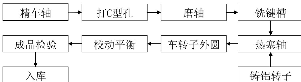
成品转子生产工艺流程图
