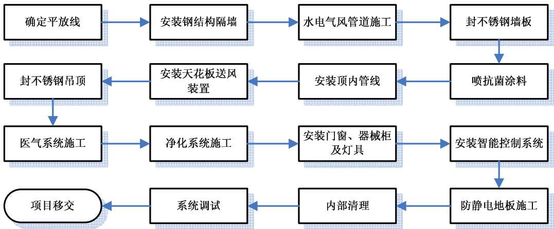
净化系统施工流程图
