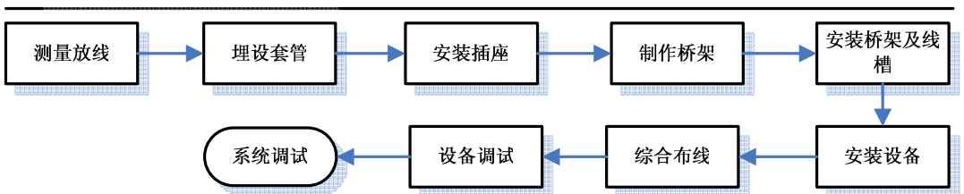
智能控制系统施工流程图
