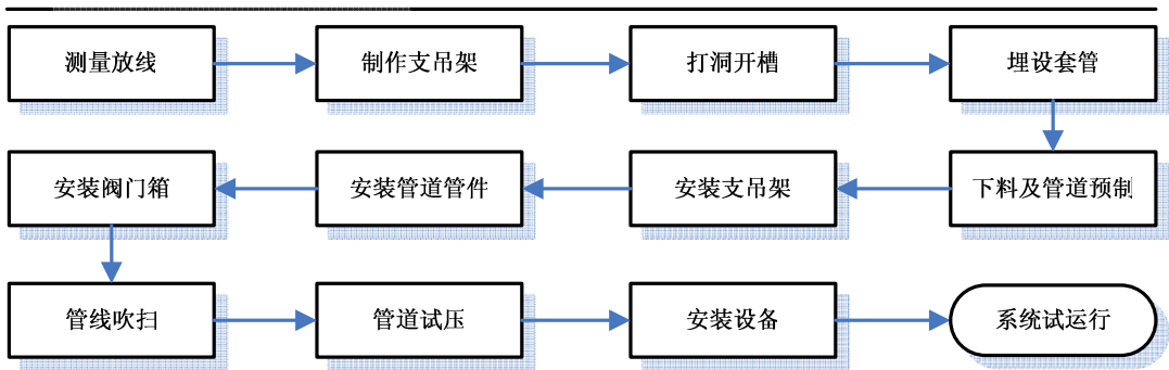
医气系统施工流程图
