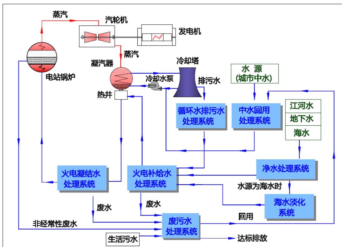
火电厂水循环系统示意图
