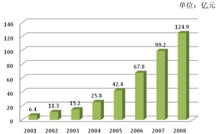
我国液压支架产值发展趋势图
