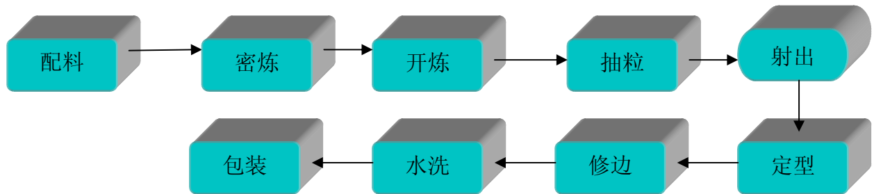
图 6-9：EVA 中底生产流程
