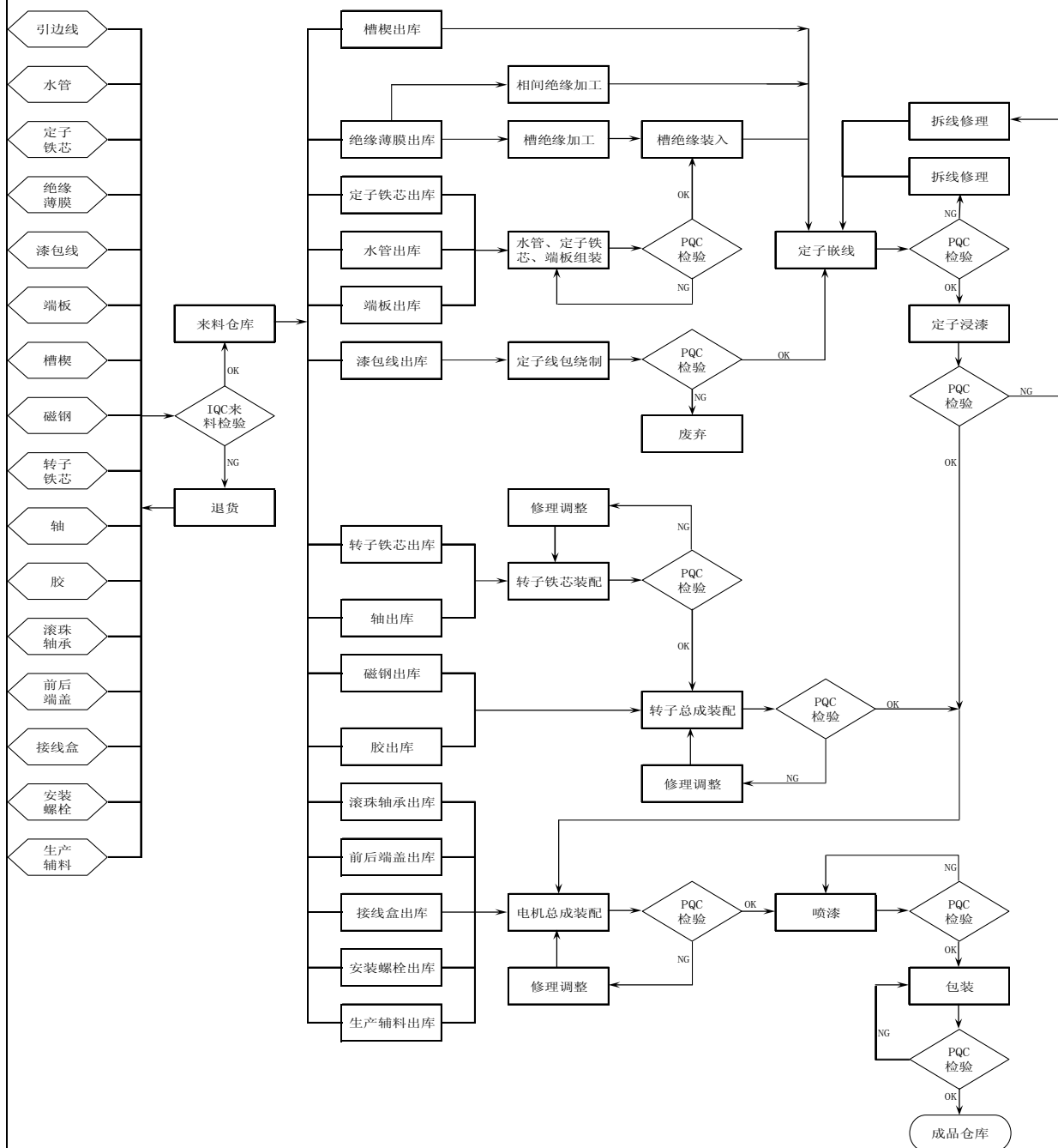
交流永磁同步电机直驱系统工艺流程图
