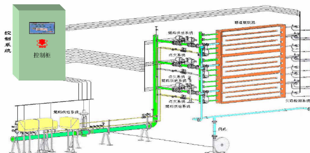
控制及管路系统示意图：
