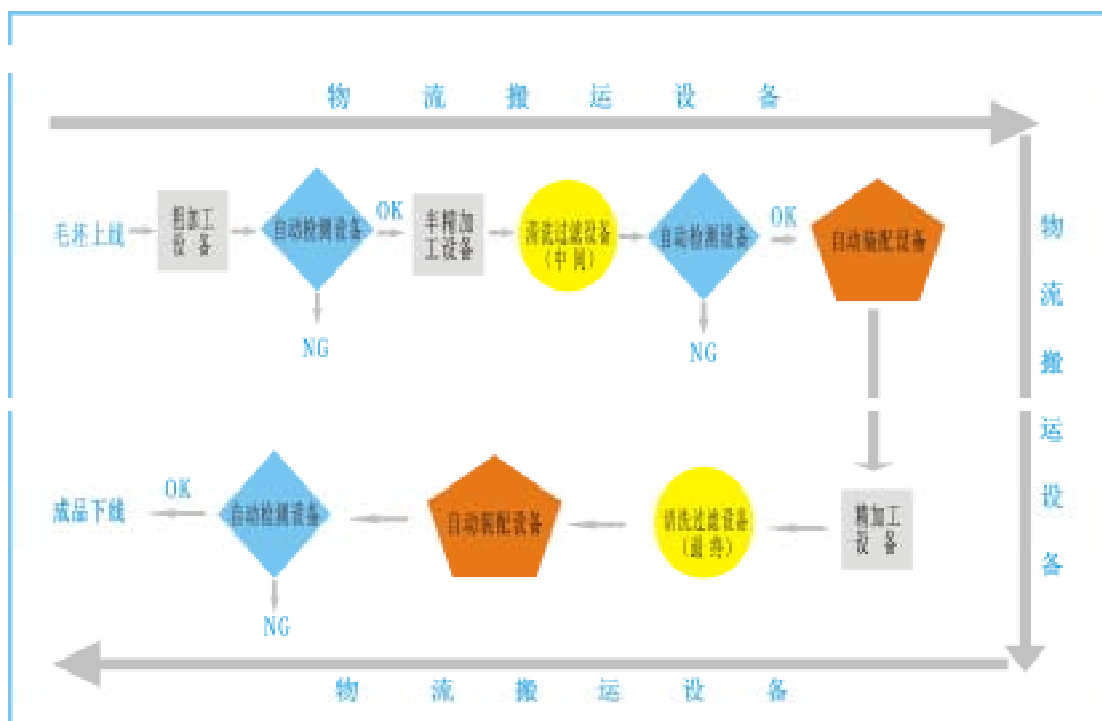
汽车零部件自动化生产线设备示意图
