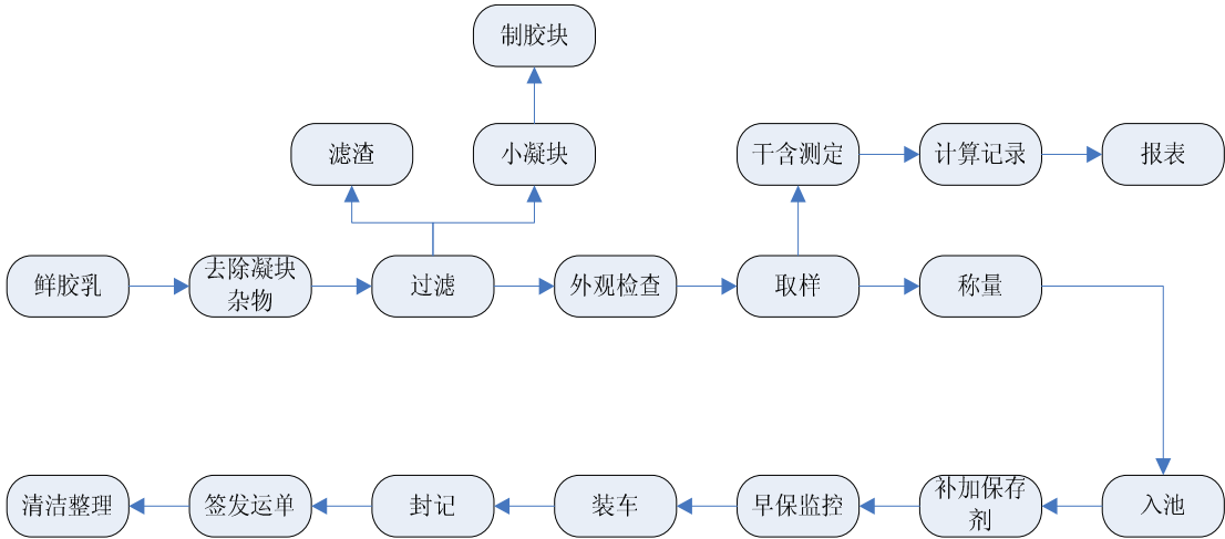
图 6.19 鲜胶乳质量控制流程
