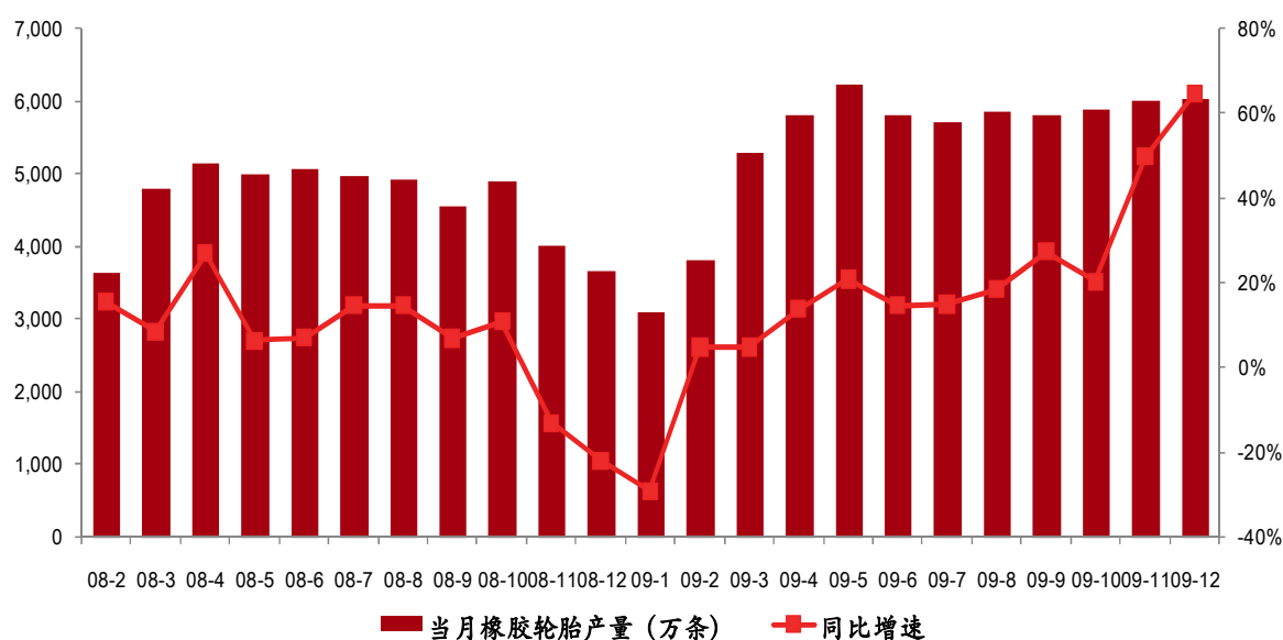
图 6.14 我国轮胎生产量
