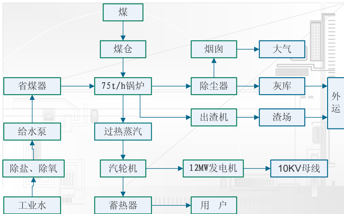
图6.19：蒸汽生产工艺流程图
