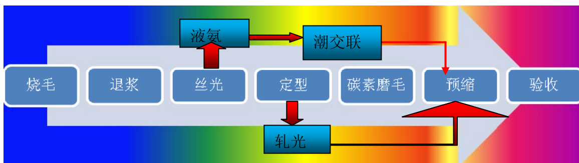
图6.15：整理工艺流程图
