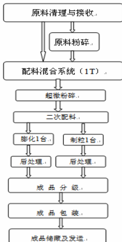
特种水产饲料生产工艺流程图
