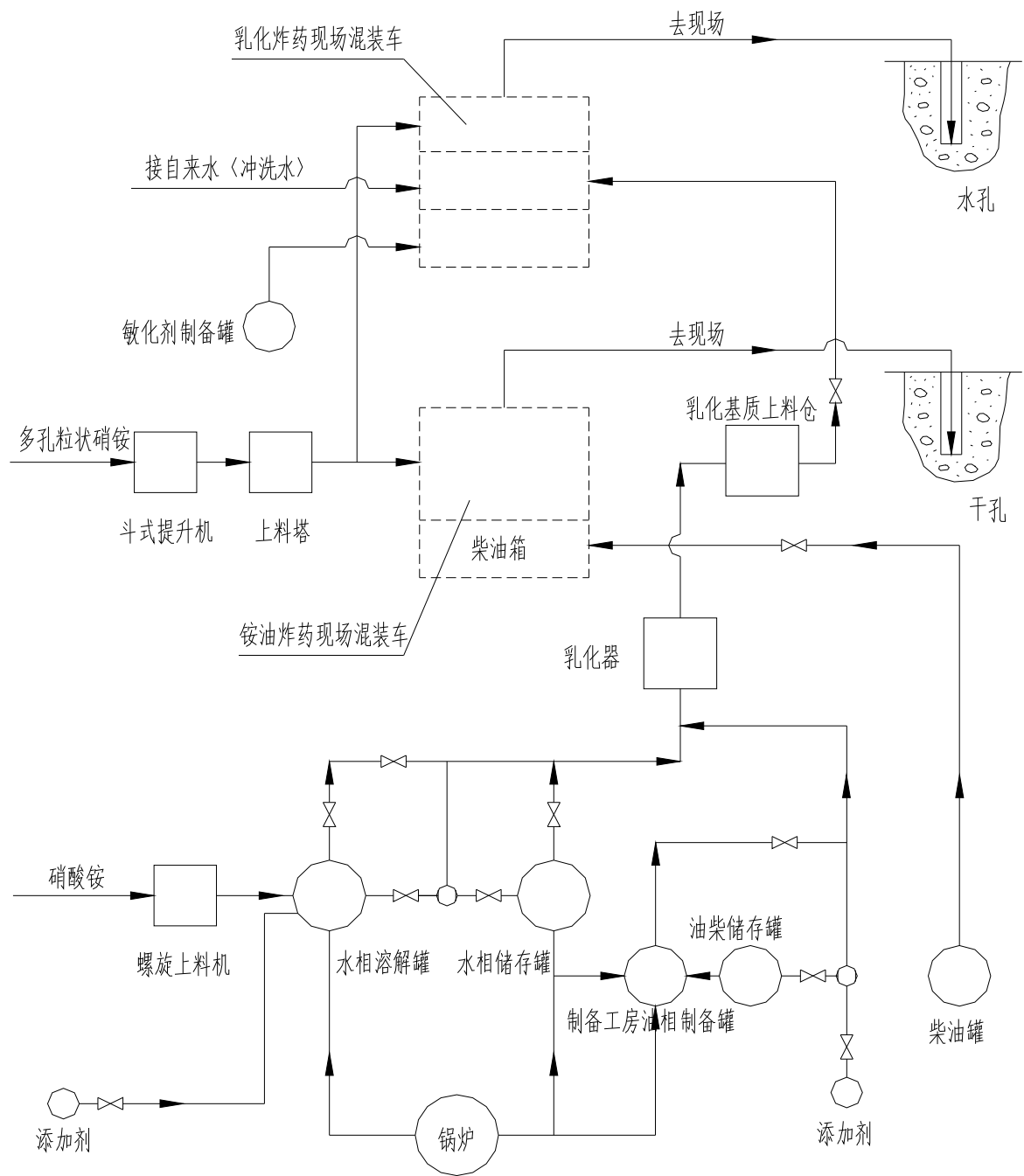
②多孔粒状铵油炸药生产工艺流程
