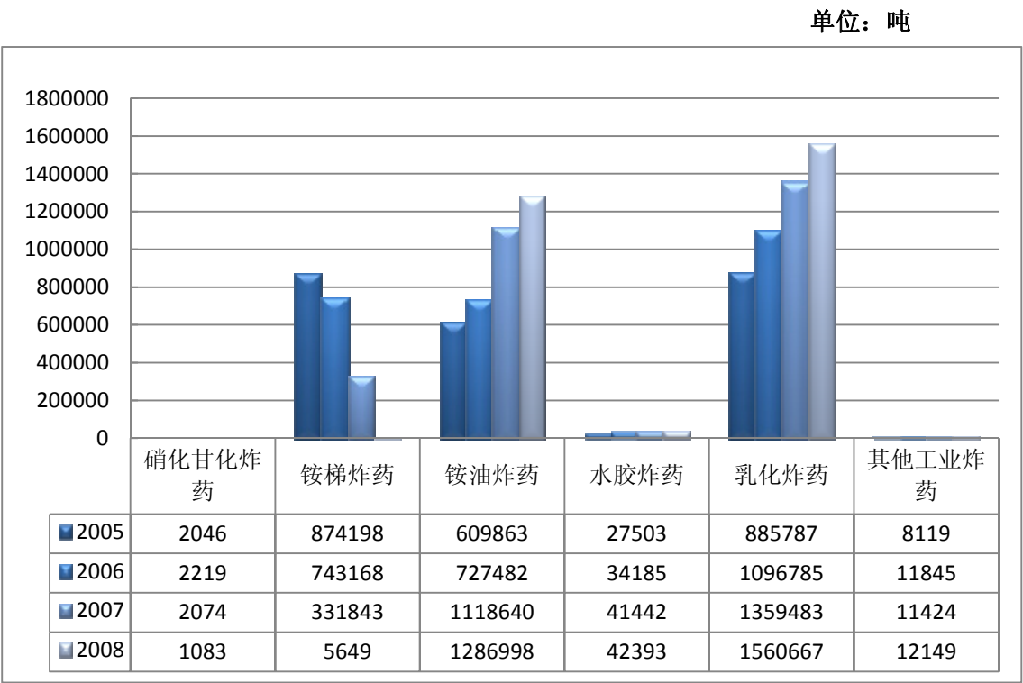
2005 年—2008 年全国不同工业炸药品种的产量变动图
