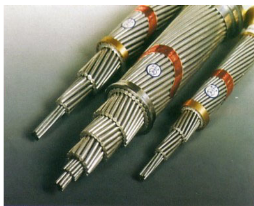
作为导线（钢芯铝绞线）的钢芯骨架
