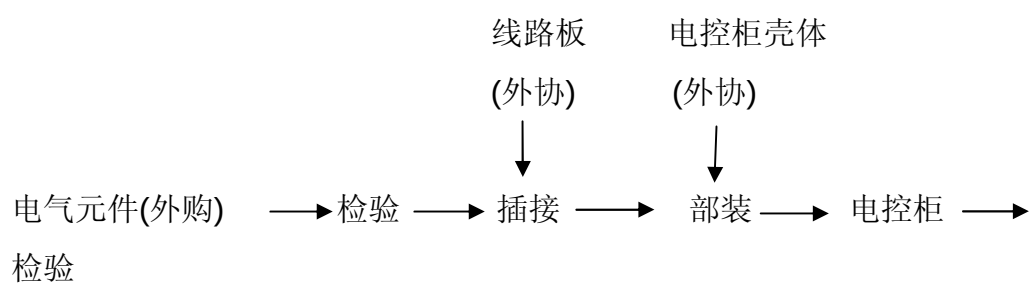
图 13-3 电控柜生产工艺流程图
