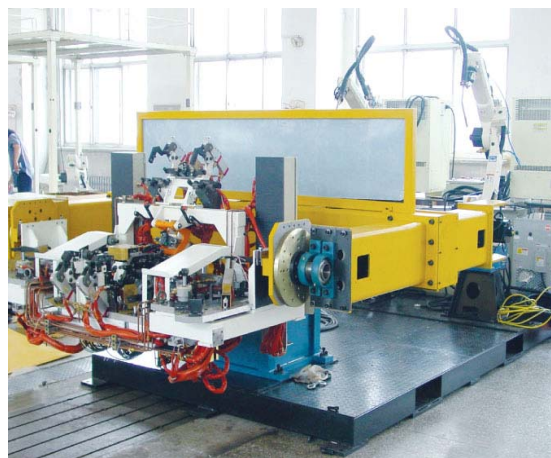
汽车座椅弧焊工作站
