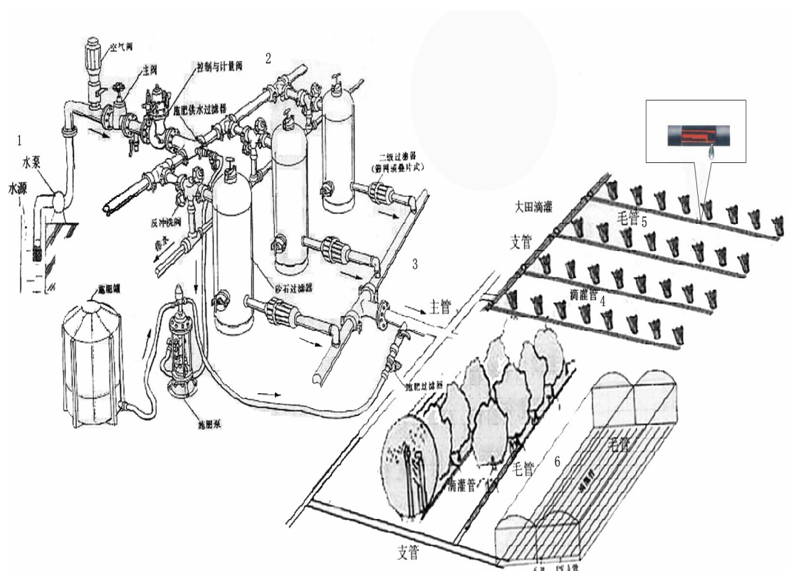
滴灌系统构成示意图：
