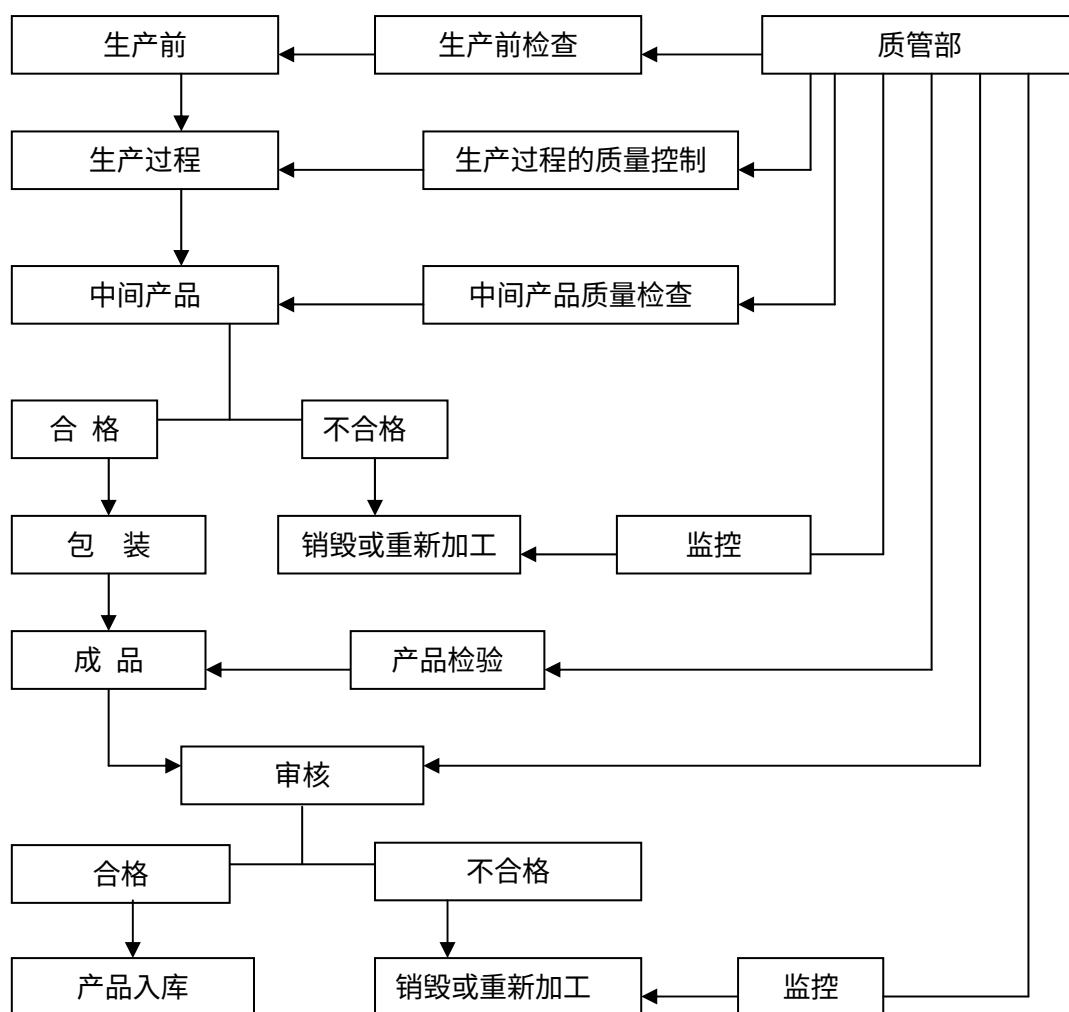
发行人生产过程质量控制流程图
