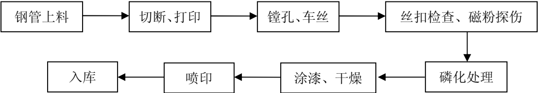
(2) 接箍加工生产线工艺流程图如下：
