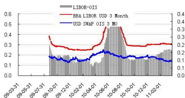
图表 20 LIBOR-OIS
