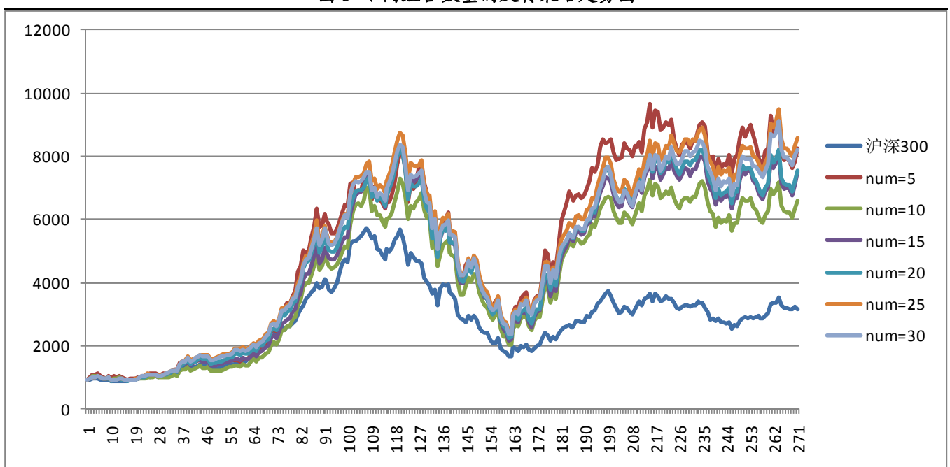
图 9 不同组合数量的反转策略走势图
