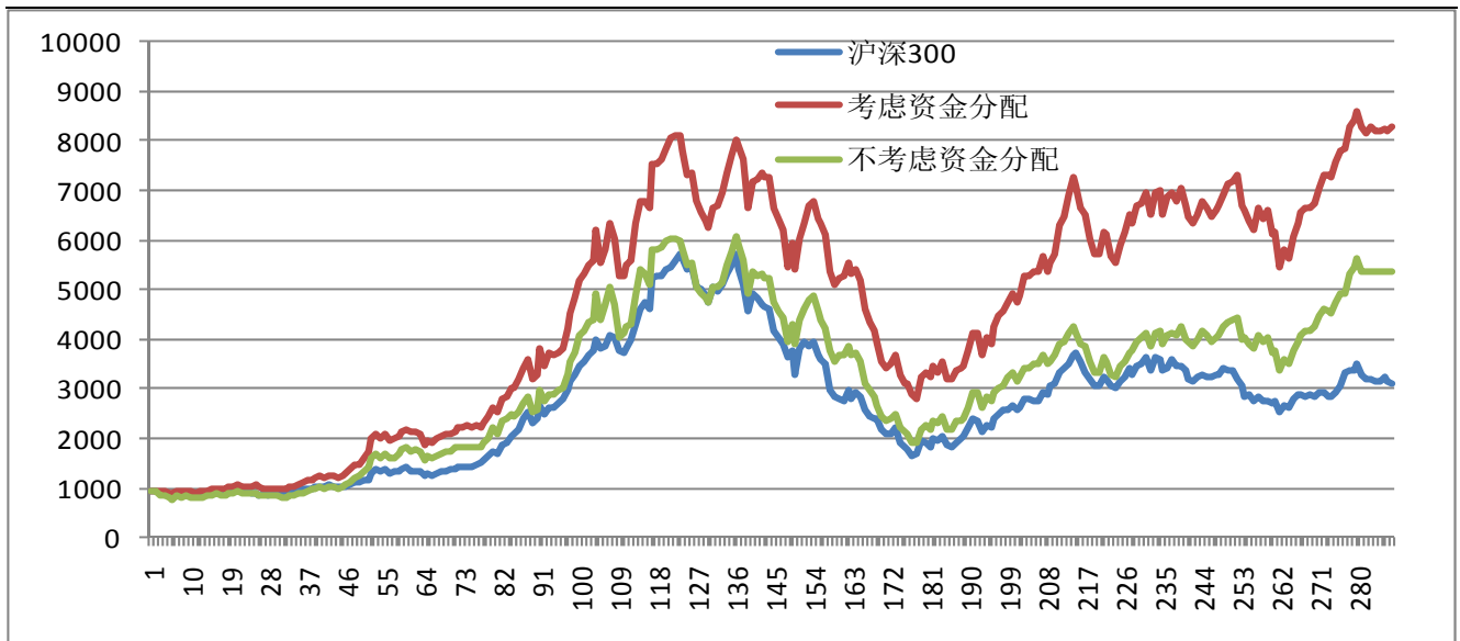
图 5 资金分配对动量策略的影响
