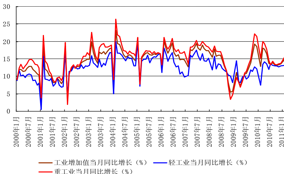
图表 4：重工业带动整体工业增加值反弹
