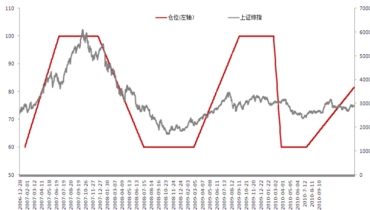
图 9： HURST 簇指数
