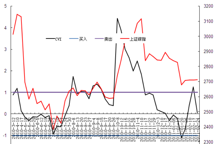
图 8： CVI 指数
