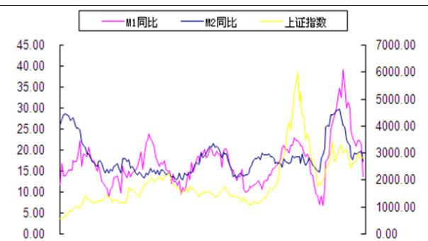
图 14: M1、M2 与股指
