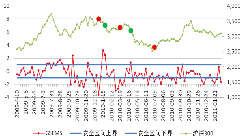
图 2: GSEMS 指标与沪深 300 指数走势对照（流通市值加权 EMS，红色圆为买点，绿色圆为卖点）
