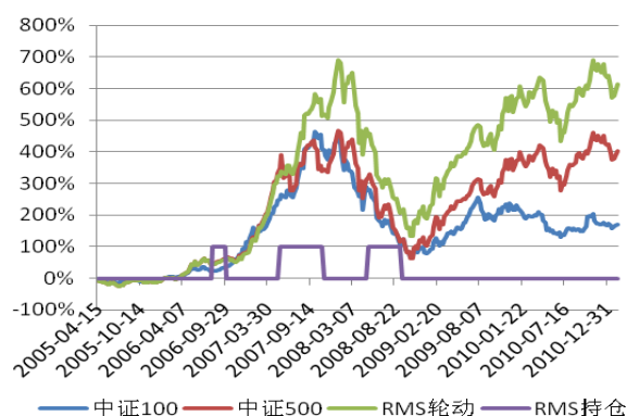
图 15: RMS 轮动策略样本内+样本外效果 (RMS 持仓=1 为持有中证 100, RMS 持仓=0 为持有中证 500)
