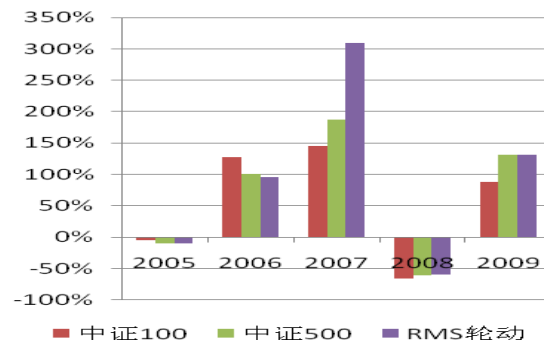
图 13: RMS 轮动策略年度收益对比 (2005-2009)
