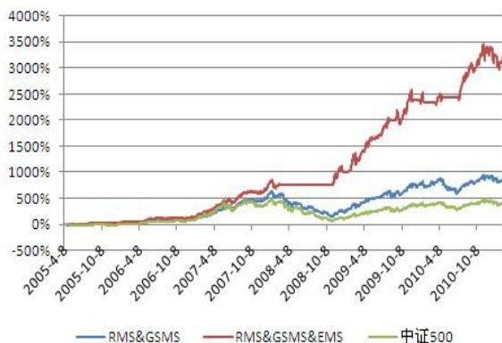
图 17: 不同策略结合后的样本内+样本外效果 (2005-4-8 至 2011-2-11)
