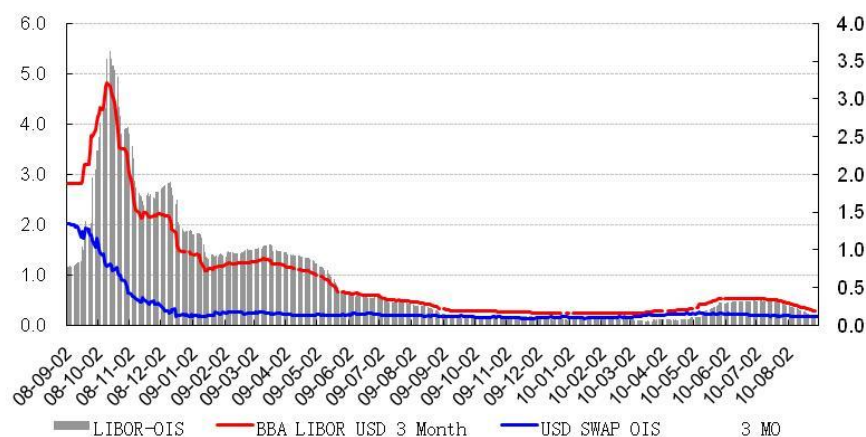
图表 12 LIBOR-OIS
