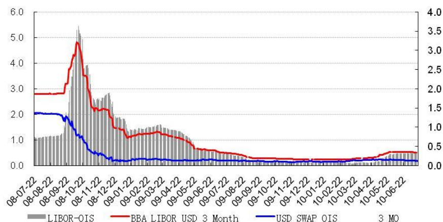
图表 12 LIBOR-OIS
