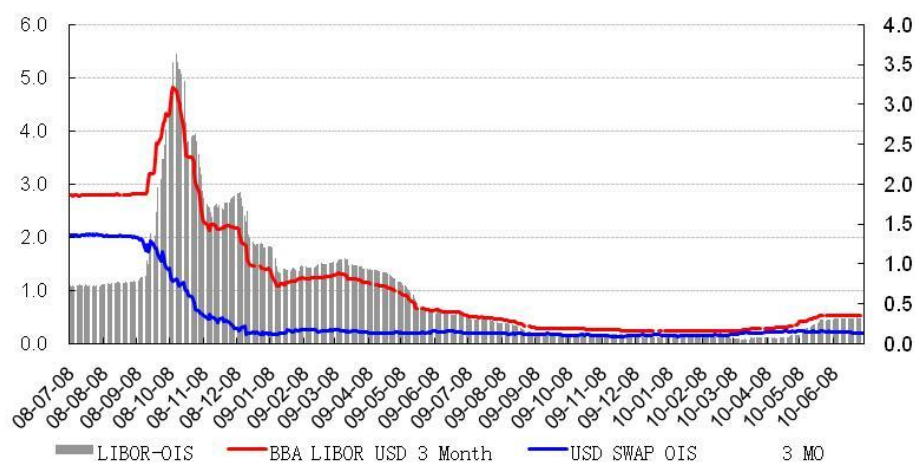
图表 12 LIBOR-OIS
