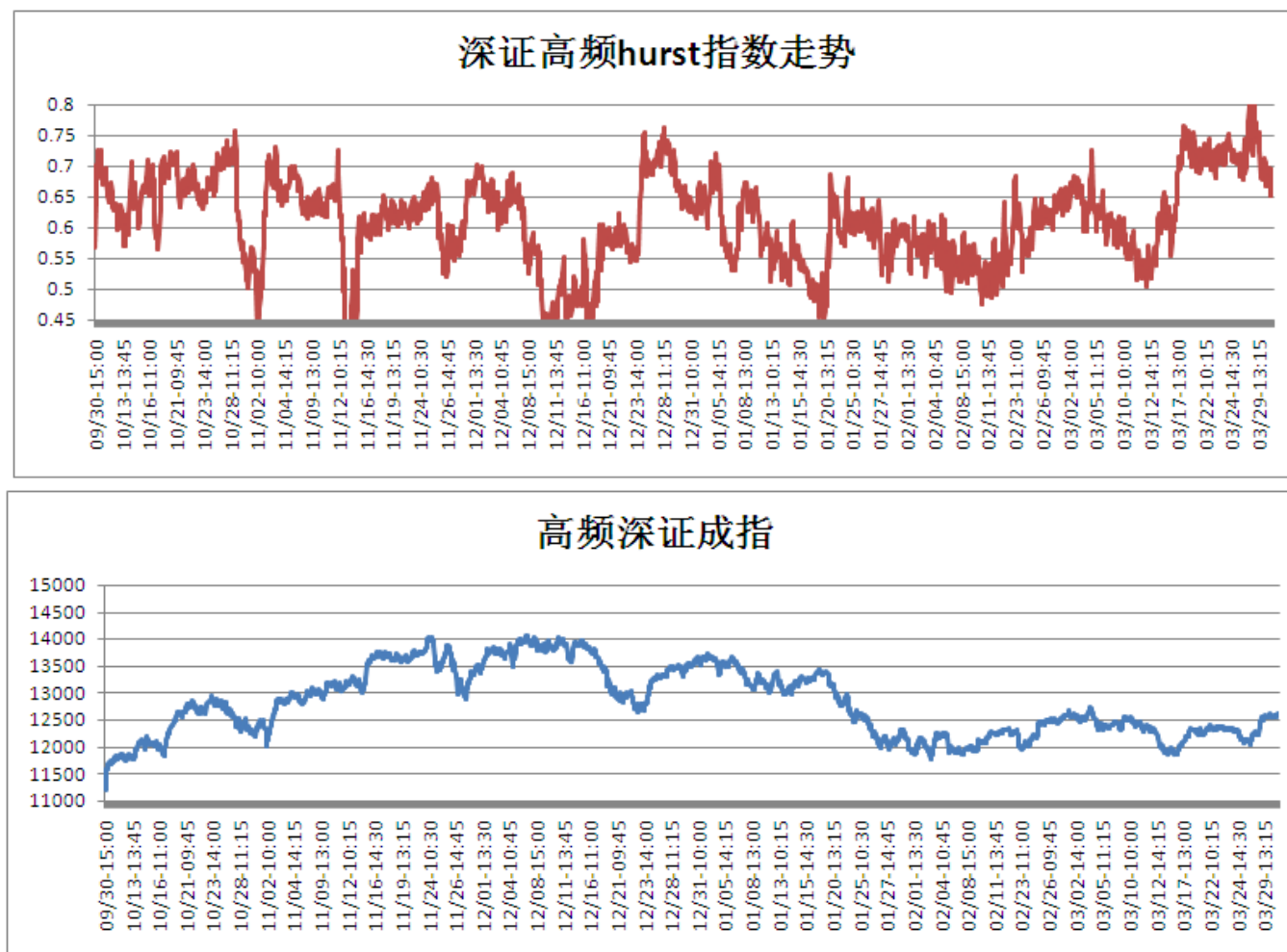
图 2 深证高频 Hurst 指数及深证成指走势
