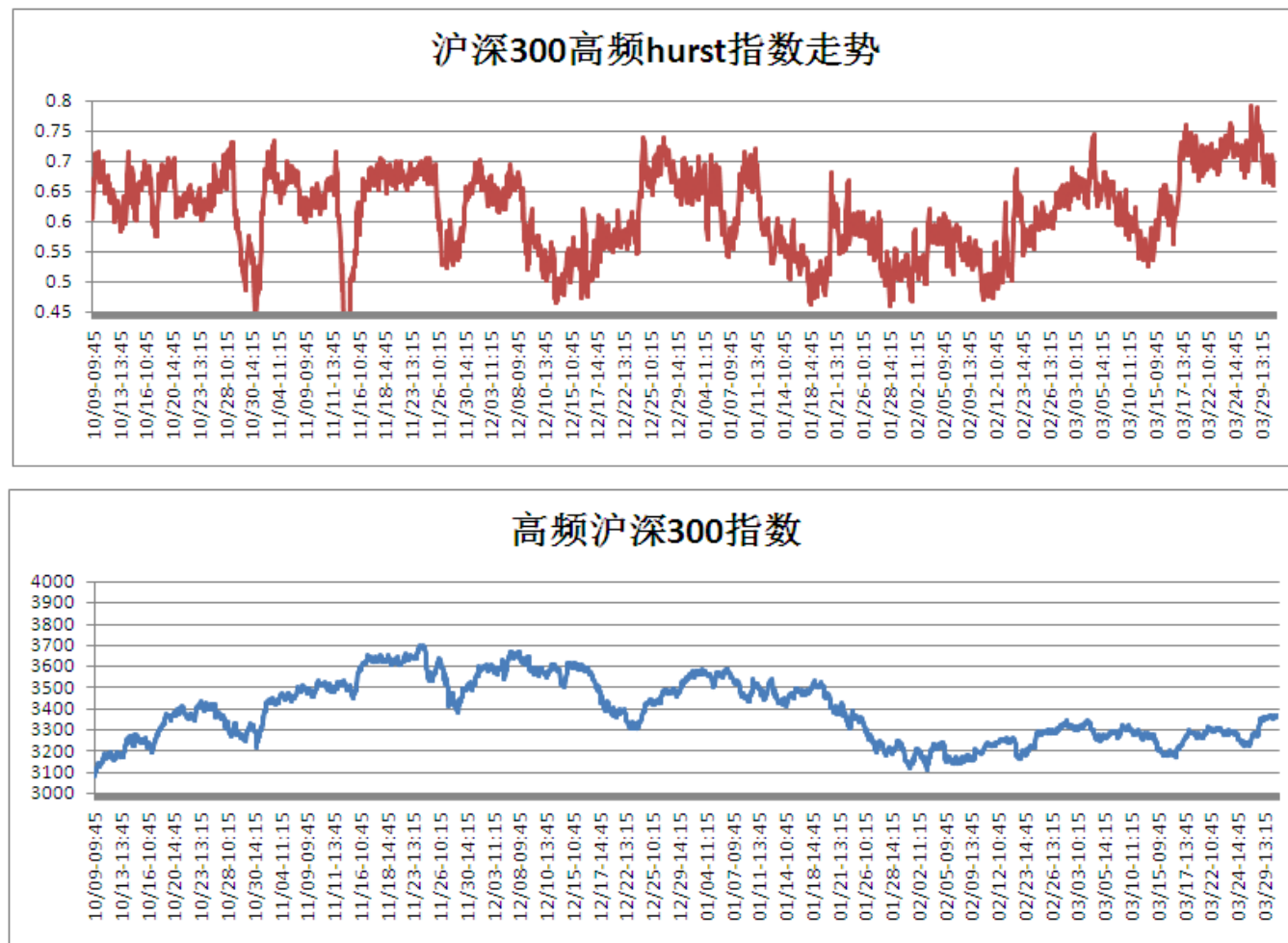
图 3 沪深 300 高频 Hurst 指数及沪深 300 走势
