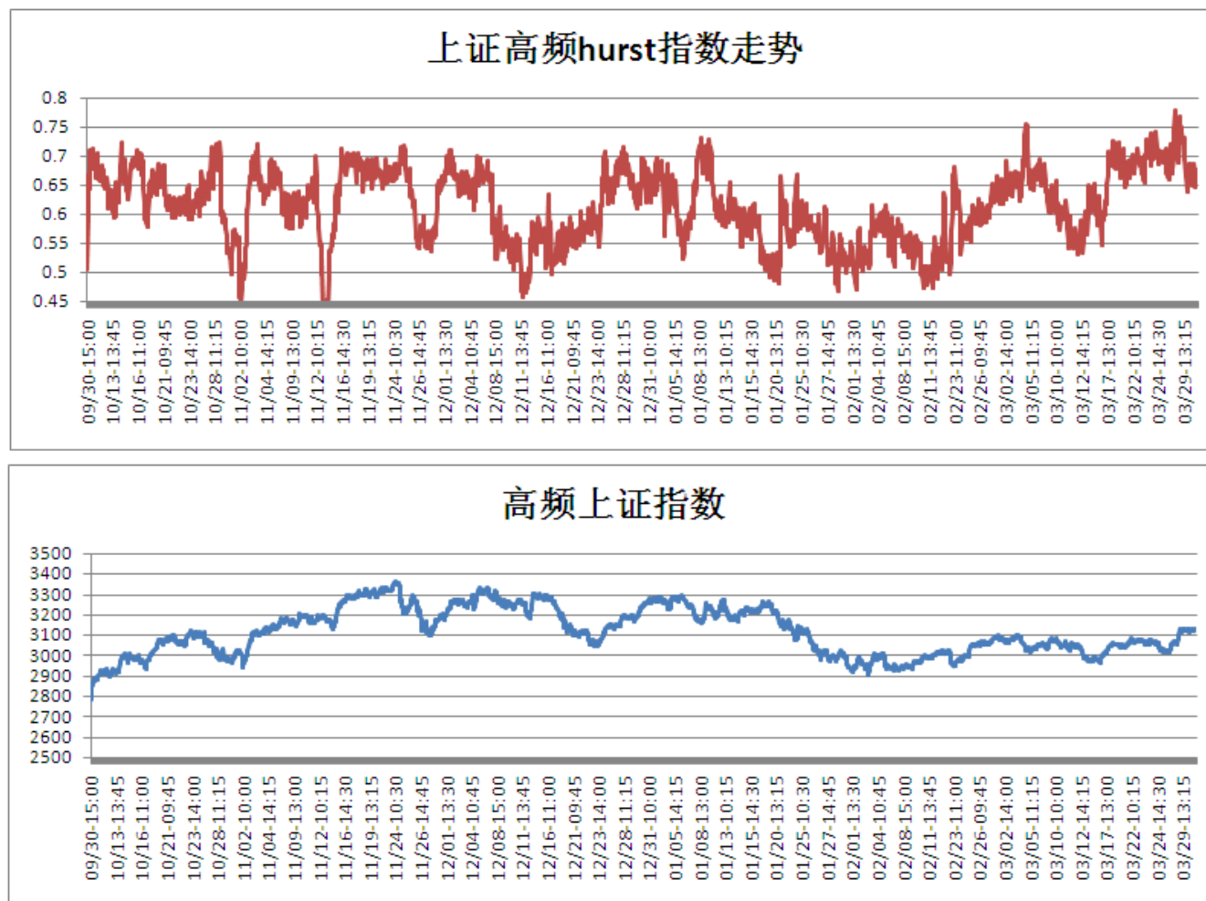
图 1 上证高频 Hurst 指数及上证指数走势
