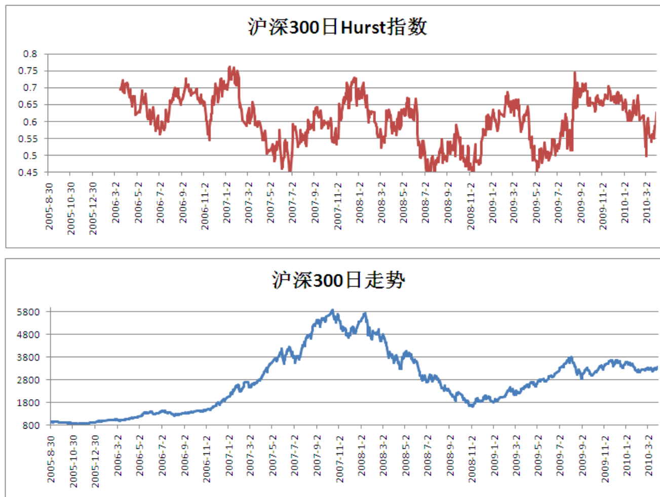
图 6 沪深 300Hurst 指数及沪深 300 指数走势（日）
