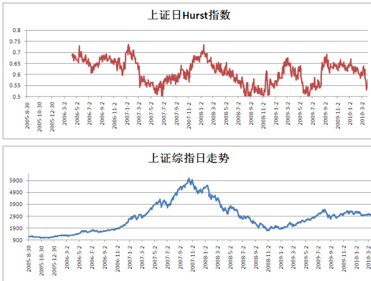
图 4 上证 Hurst 指数及上证指数走势（日）
