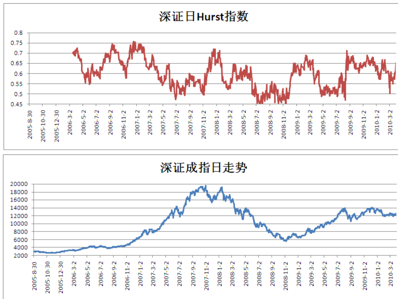
图 5 深证 Hurst 指数及深证指数走势（日）
