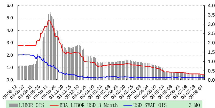
图表 10 LIBOR-OIS
