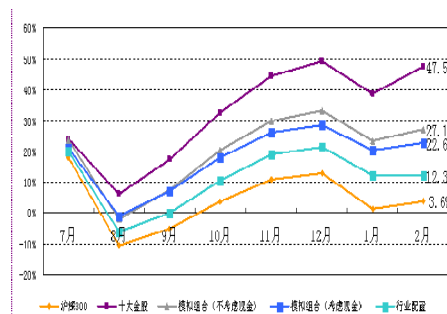
光大策略行业配置累积收益率
