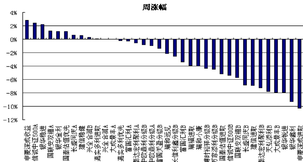
图 1：周表现排序
