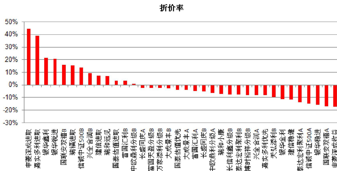
图 2：折价率排序
