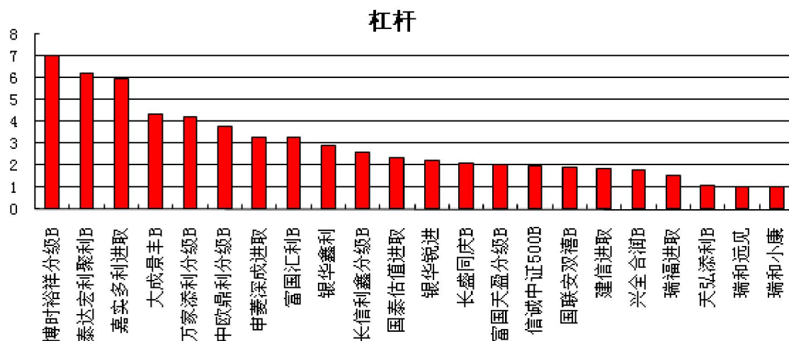
图 5：杠杆
