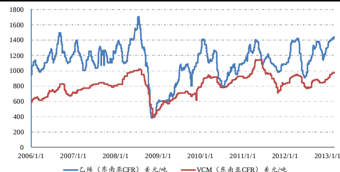
图2：乙烯、VCM东南亚到岸价
