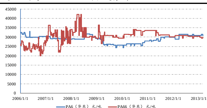
图2：国内 PA6、PA66价格走势图
