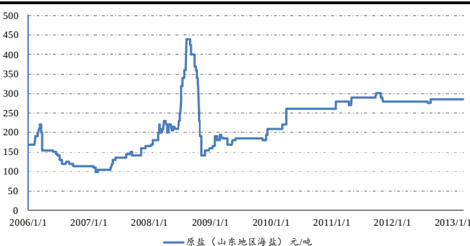
图2：山东潍坊地区原盐价格
