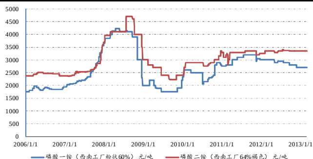
图3：国内磷酸一铵、二铵价格
