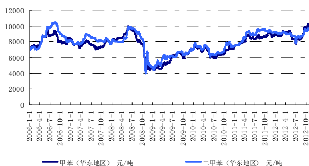
图1：国内二甲苯价格
