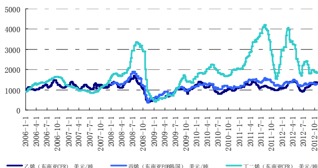
图2: 东南亚乙烯、丙烯、丁二烯到岸价
