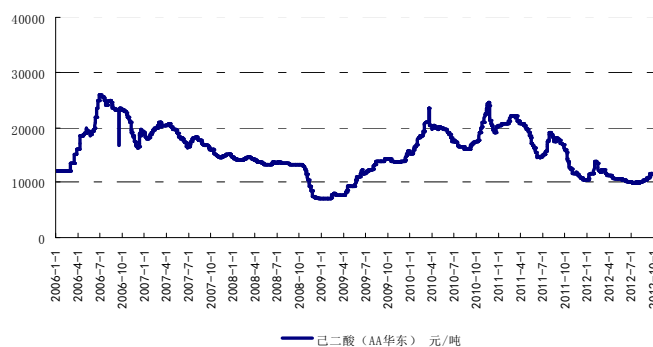
图2：国内己二酸价格走势
