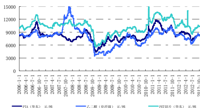
图1: PTA、MEG、PET切片价格
