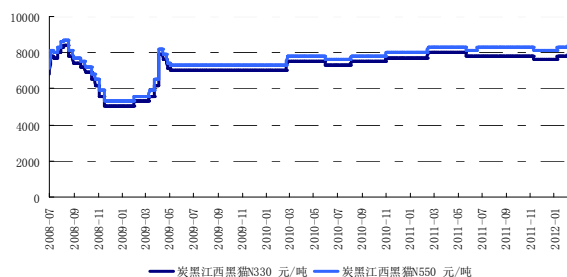
图2：炭黑价格
