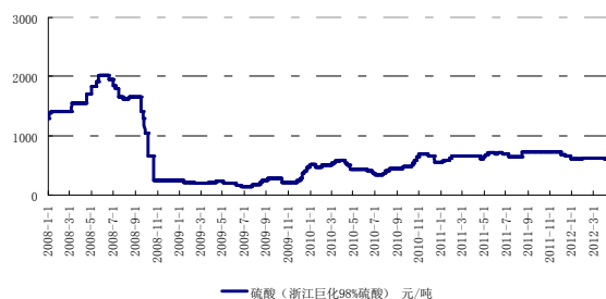
图1：硫酸价格
