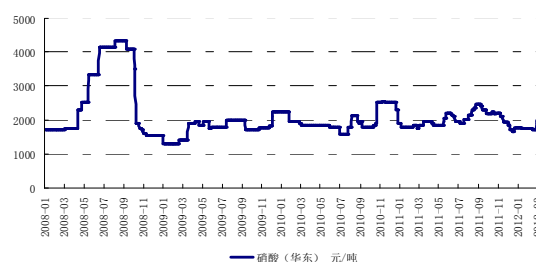
图2: 硝酸价格
