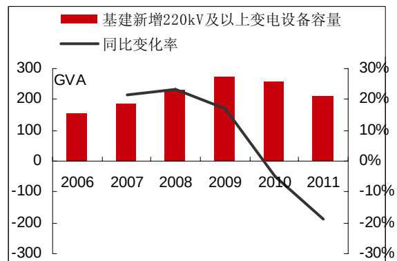
图 2: 2006~2011 年我国 220kV 及以上输电主网新增变电容量统计
