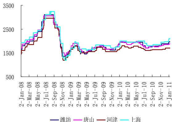
图 8：焦炭价格走势图
