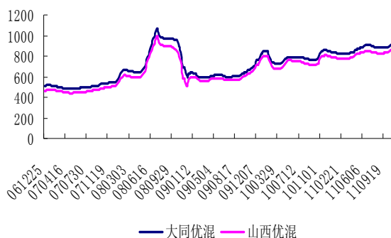
图 1：大同优混和山西优混走势图
