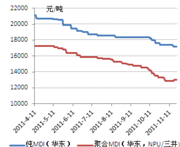
图 40: 国内 MDI 产品价格
