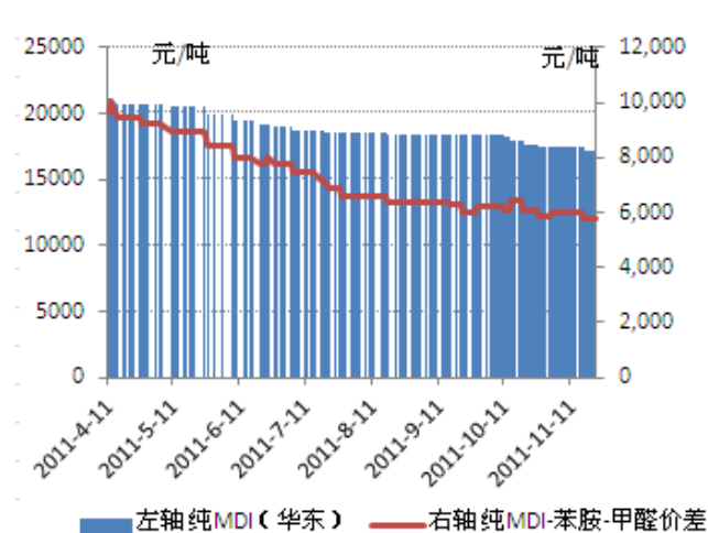
图 41: MDI 价格及价差
