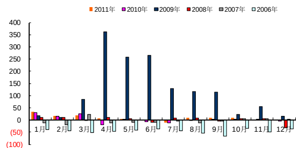
图 9：中国原铝净进口（2006-2011）KT
