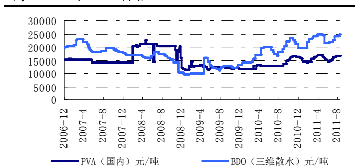
图1：PVA、BDO价格
