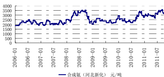
图1：合成氨价格
