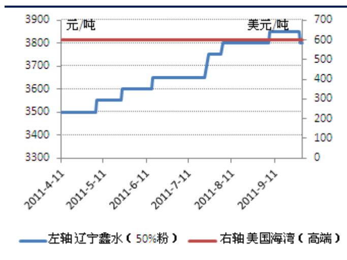
图 26: 国内外硫酸钾价格
