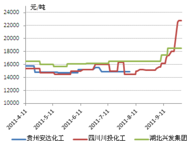
图 30: 国内黄磷价格
