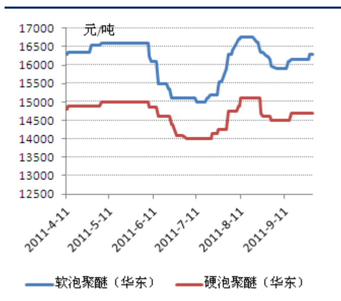
图 44: 国内软泡聚醚和硬泡聚醚产品价格
