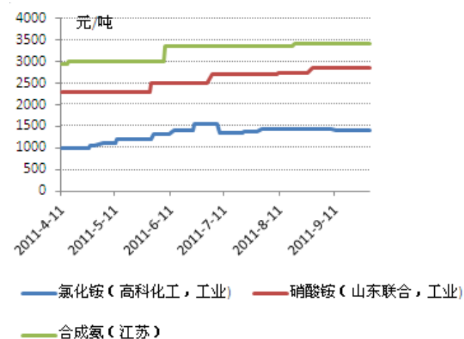
图 22: 氮肥相关产品价格
