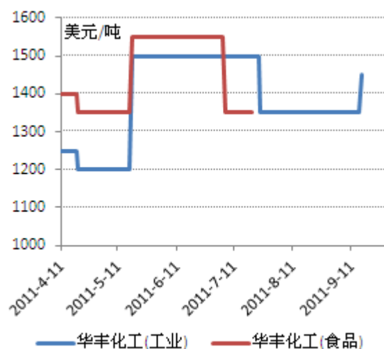
图 31: 国内三聚磷酸钠价格
