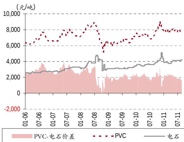
图表 41. 电石法 PVC 价差图
