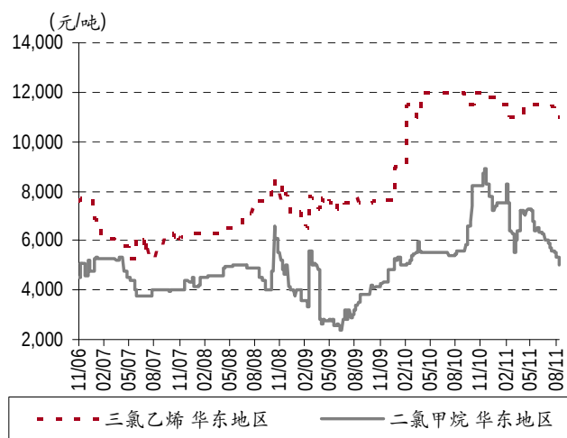
图表 57. 三氯乙烯和二氯甲烷价格
