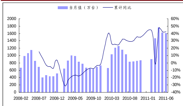
图 2: 空调产量
