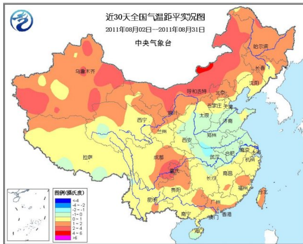
图 3：气温变化
