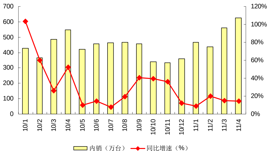
图表 冰箱内销及同比增速
