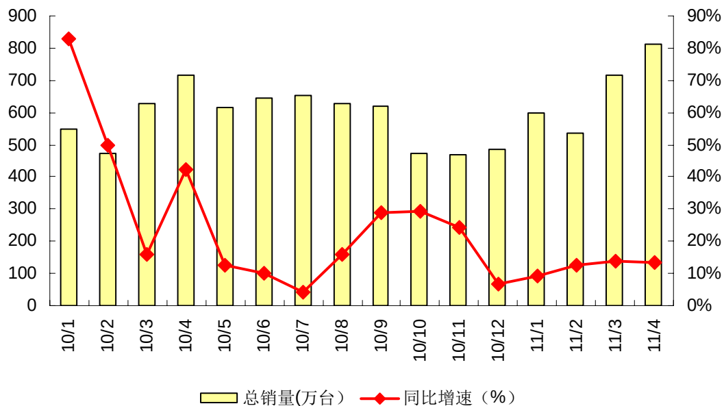
图表 冰箱总销量及同比增速
