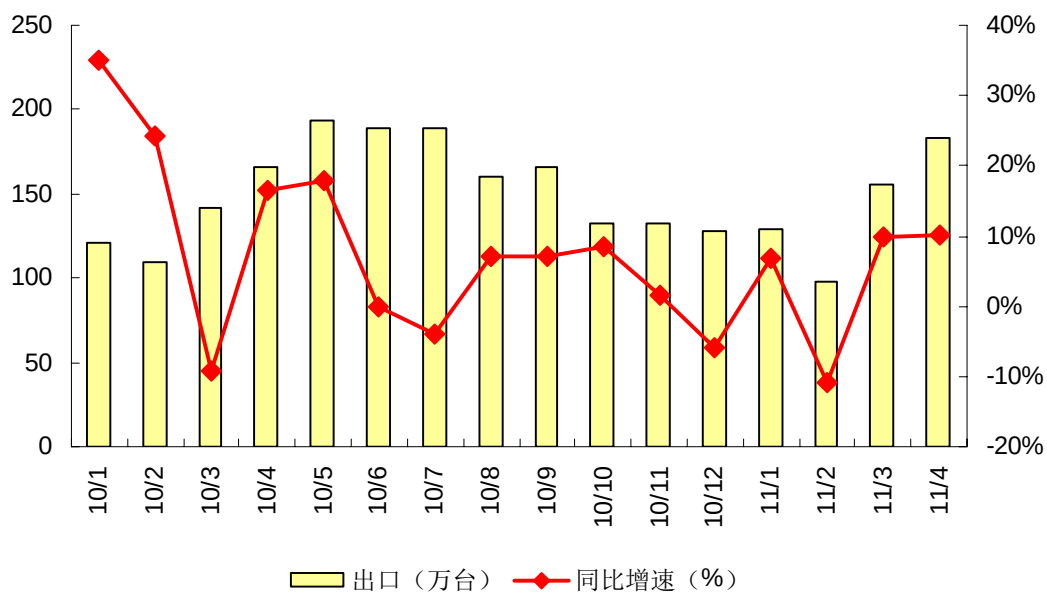
图表 冰箱出口销量及同比增速
