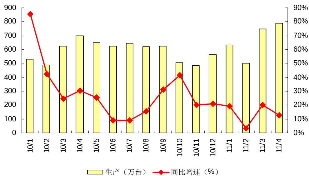
图表 冰箱产量及同比增速
